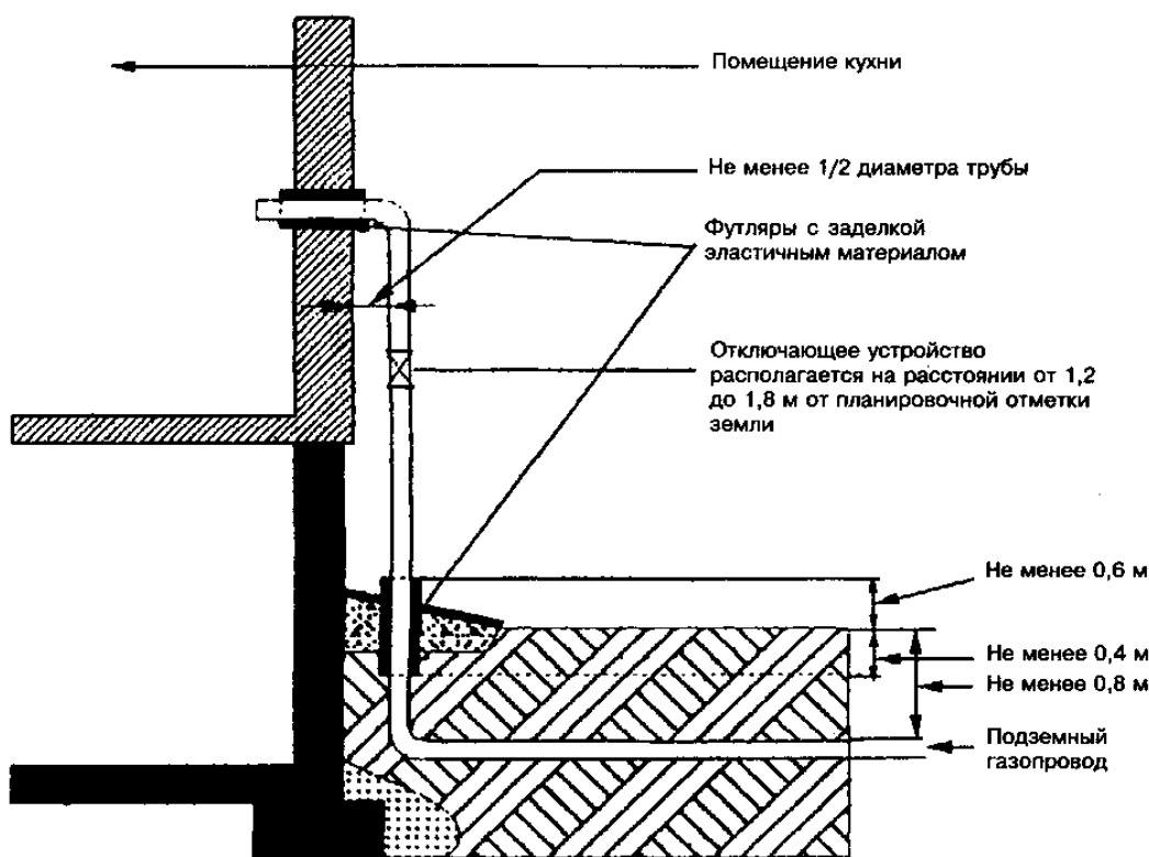
Рисунок 9.1 — Газовый ввод
