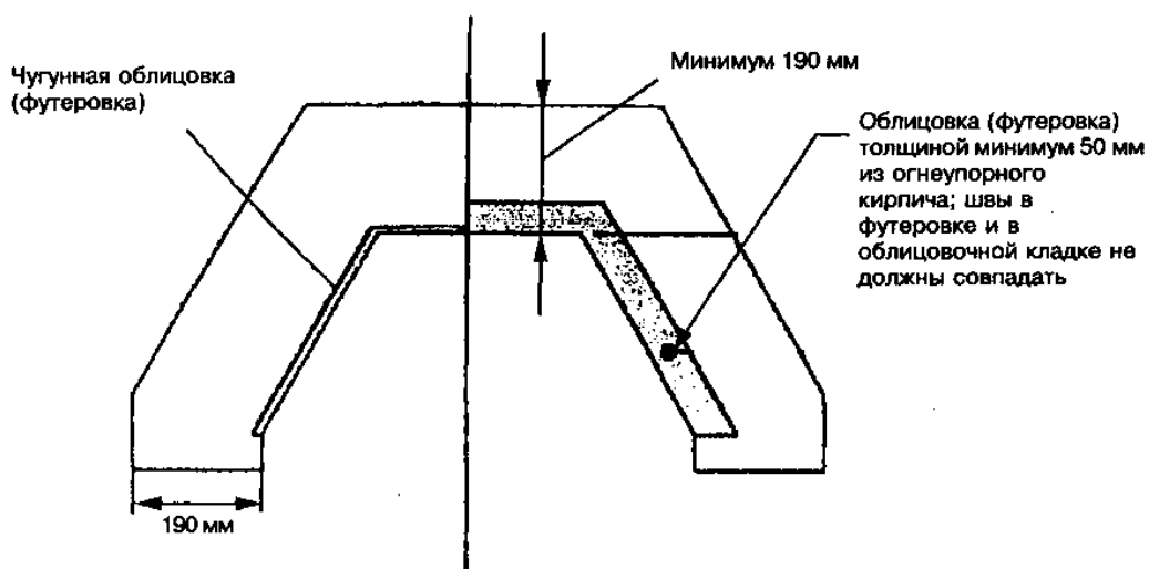
Рисунок 7.5 — Футеровка камина
